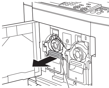
Poignée du tambour
