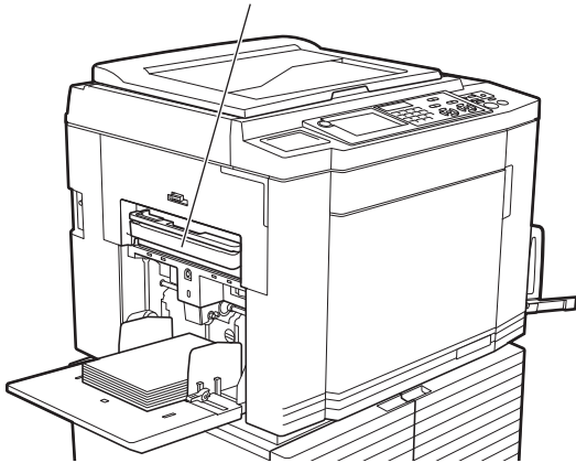
Boîte de récupération des masters du tambour 2
